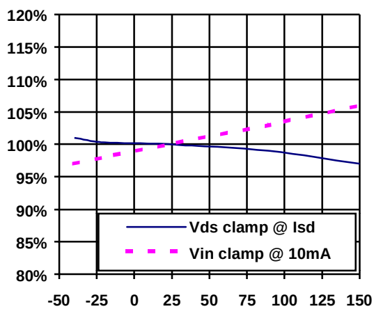
Figure 19 - Vin clamp1 & Vin clamp2 (%) Vs Tj (°C)
