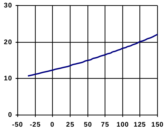
Figure 20 - Iqc (μA) vs Tj (°C)
