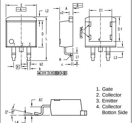
TO-263 AB
