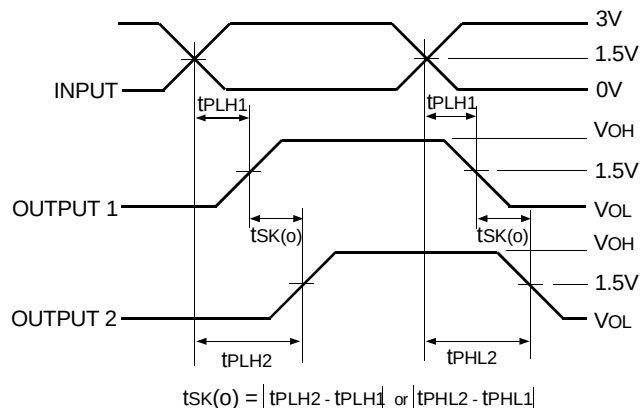
Output Skew
