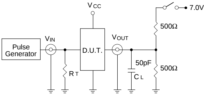
2577 drw 06
