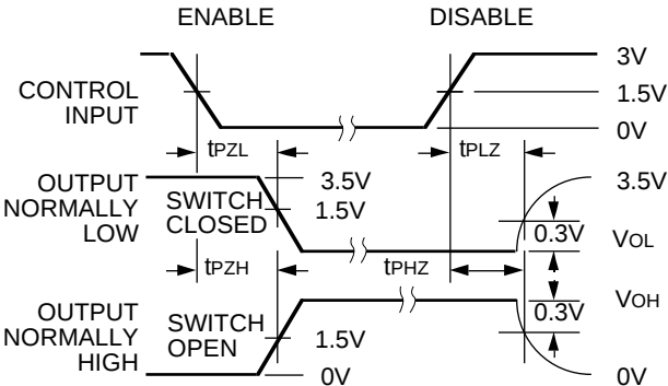
2577 drw 09
