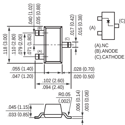
SOT-23
