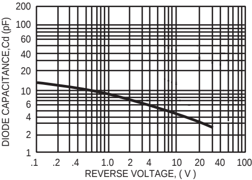
FIG. 2 - DIODE CAPACITANCE
