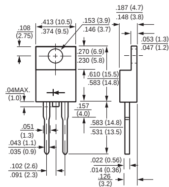
TO-220A
