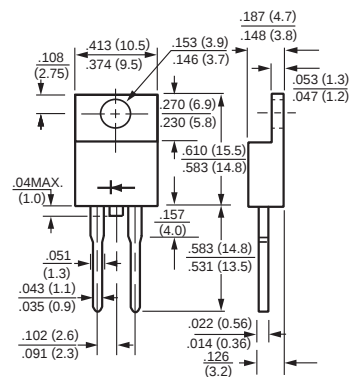
TO-220A
