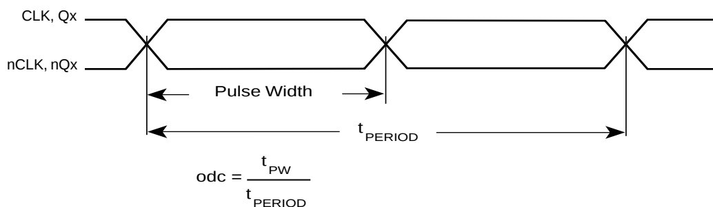
FIGURE 7 - odc & t_{PERIOD}
