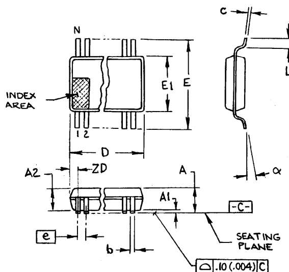
150 mil SSOP
