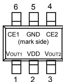
SOT-23-6
