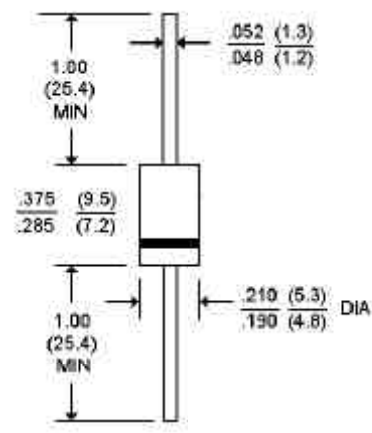
DO-201AD
