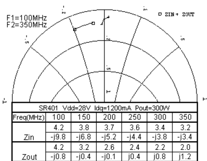
Zin Zout
