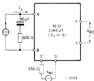
Fig. 4 – Sidetone
