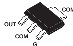
SOT-223 ACS108-5SN
