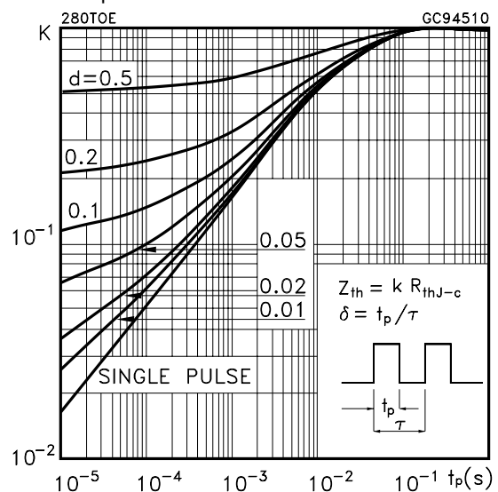
Thermal Impedance
