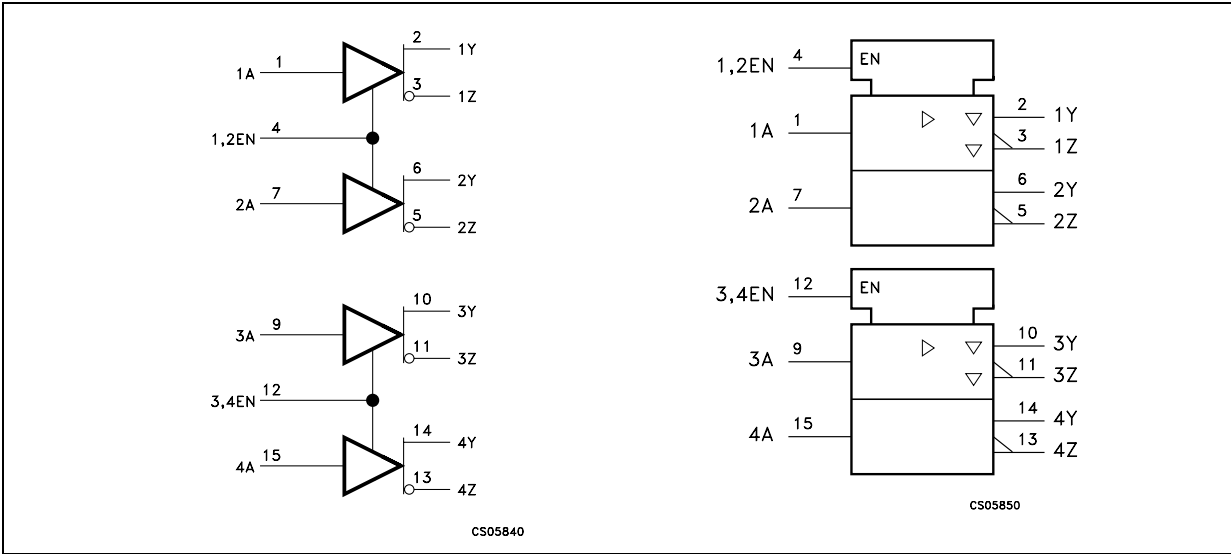
STLVDS31 TRUTH TABLE
