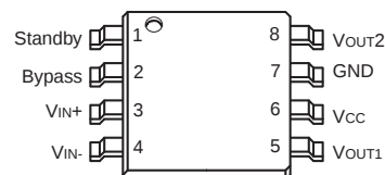
TS4871IST - MiniSO8
