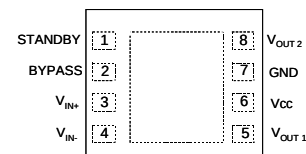
TS4871IQT - DFN8
