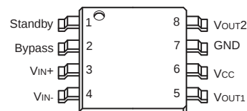
TS4871IQT - DFN8
