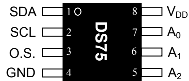
DS75U — μMAX
