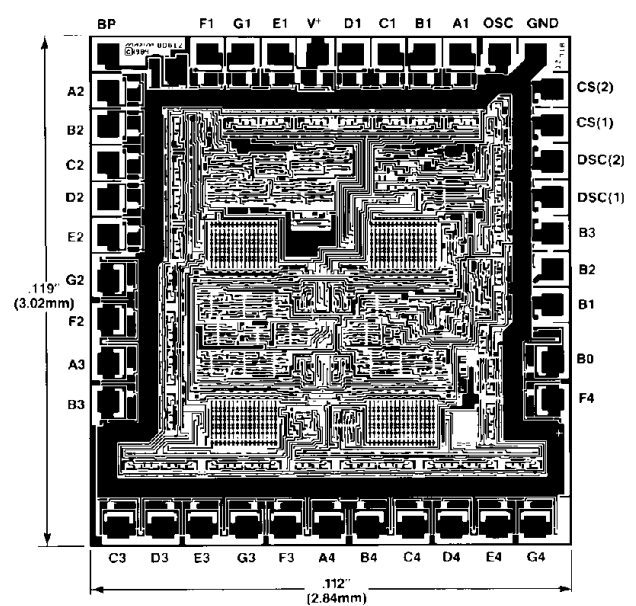
ICM7211M, 7211AM
