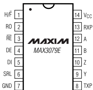
DIP/SO
