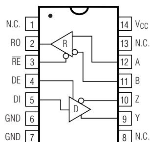
DIP/SO
