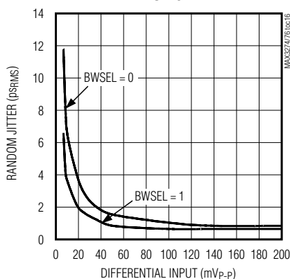
RANDOM JITTER
