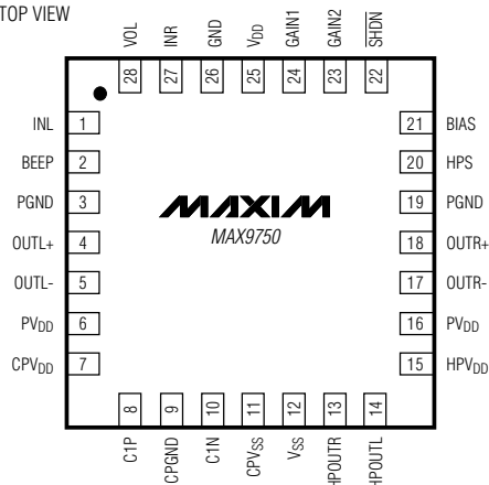
THIN QFN
