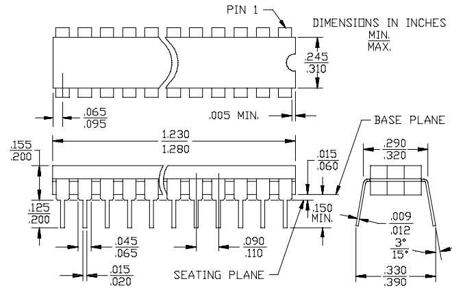
24-Lead (300-Mil) CDIP D14 MIL-STD-1835 D- 9 Config.A
