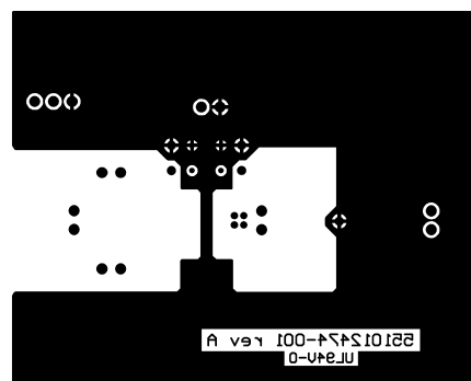
Figure 44. Bottom Layer
