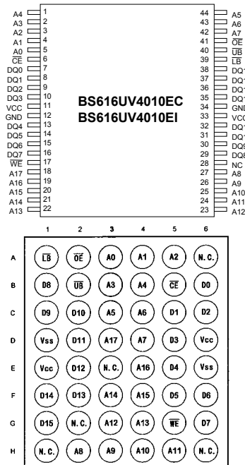
48-ball CSP - Top View
