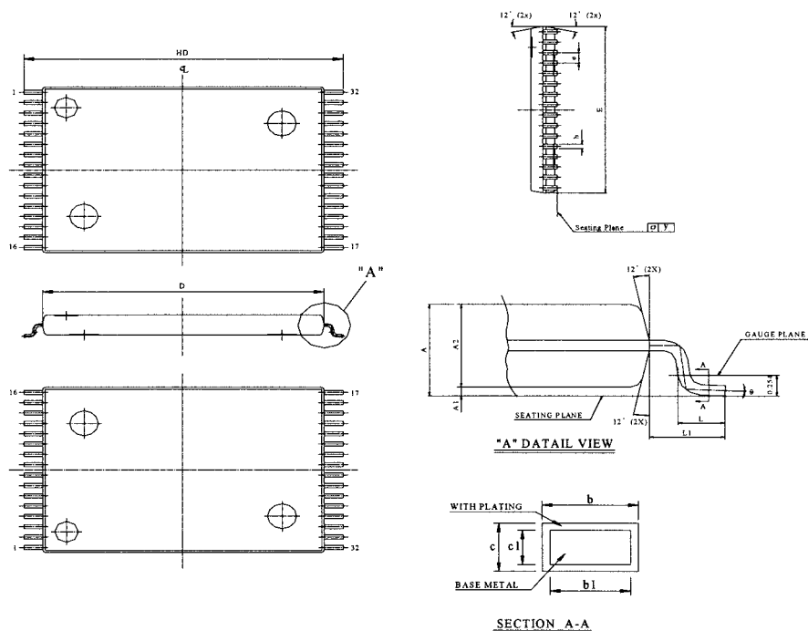
STSOP - 32
