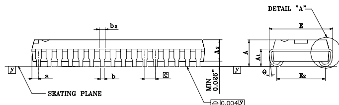
SOJ - 32
