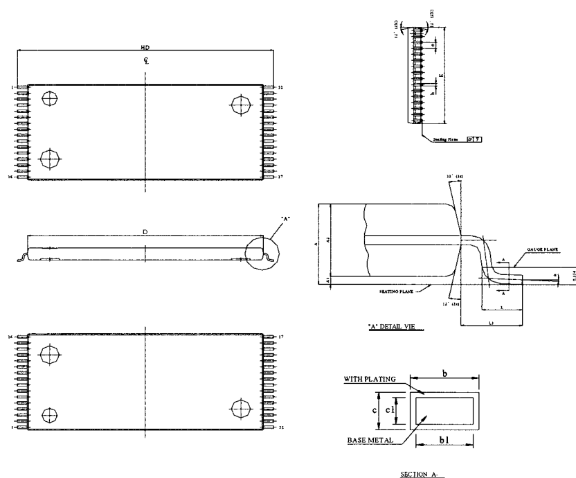
TSOP - 32
