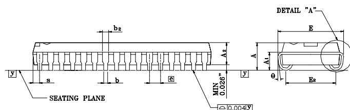
SOJ - 32
