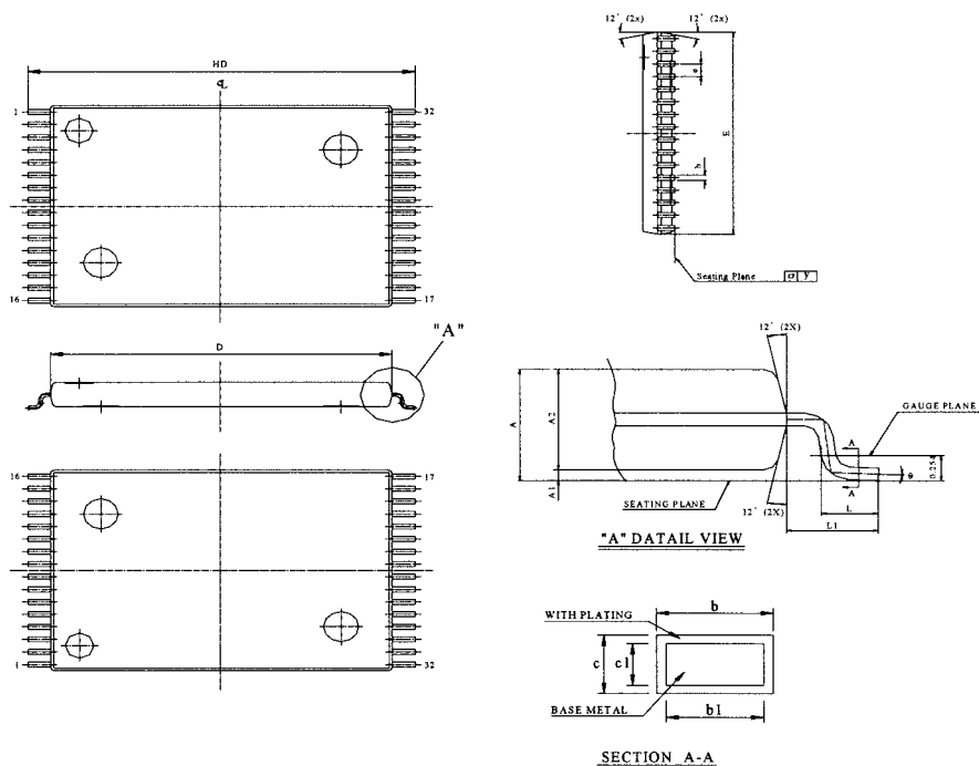
STSOP - 32
