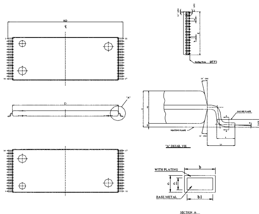
TSOP - 32
