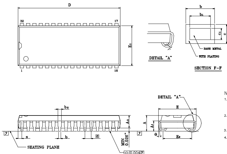
SOJ - 32
