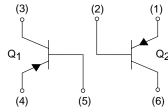
MBT3906DW1T1
