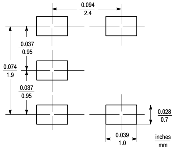
THIN SOT-23-5
