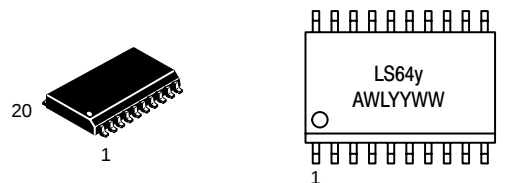
SOIC–20 DW SUFFIX CASE 751D
