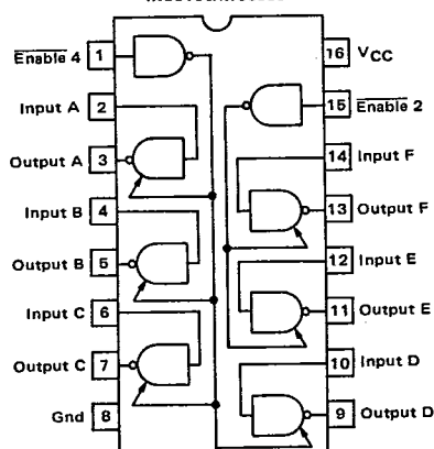
MC8T98/MC6888
