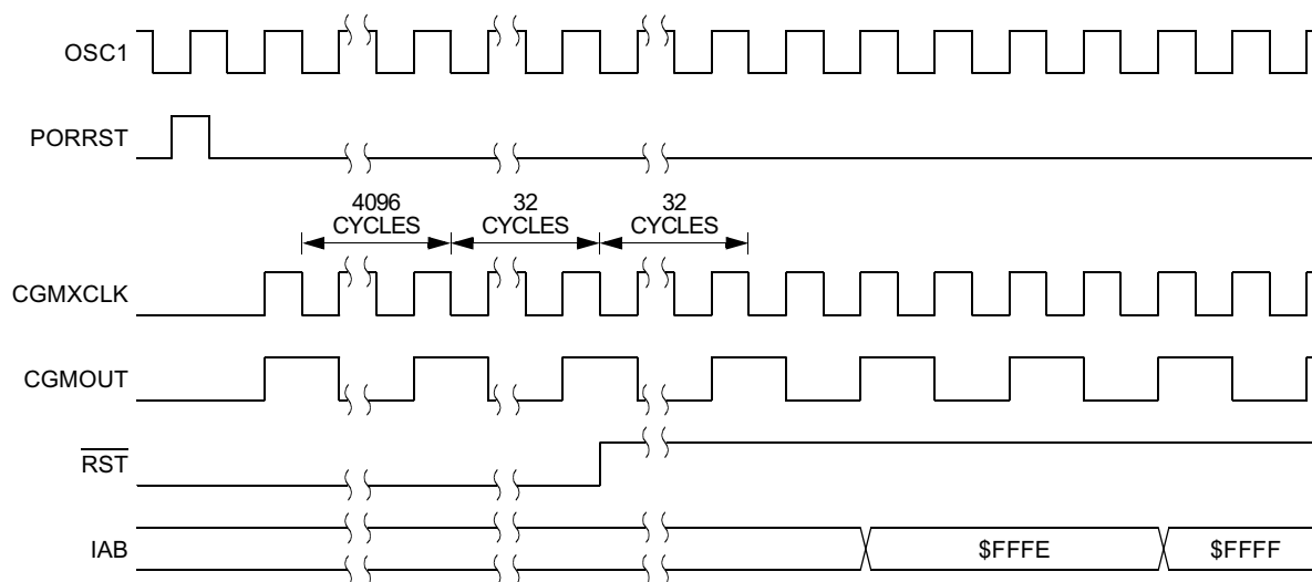
Figure 19-7. POR Recovery
