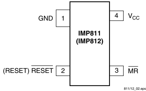
SOT143
