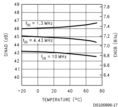
SINAD & ENOB vs Temp & f_{IN}
