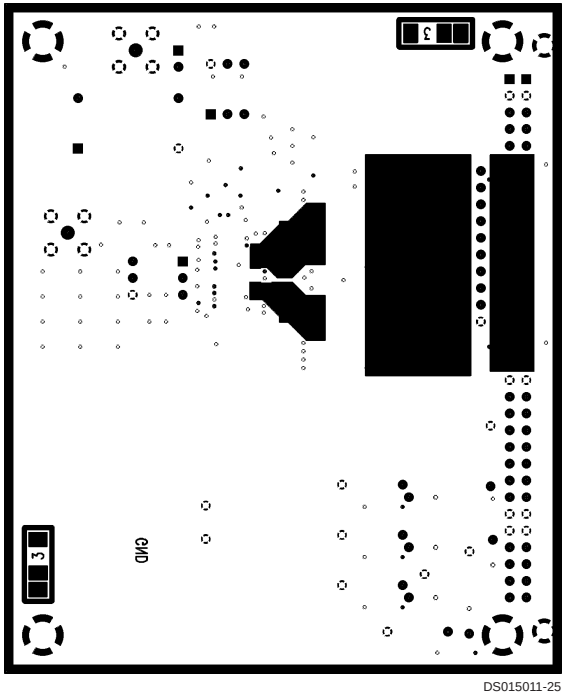
CLC730079 Layer 3
