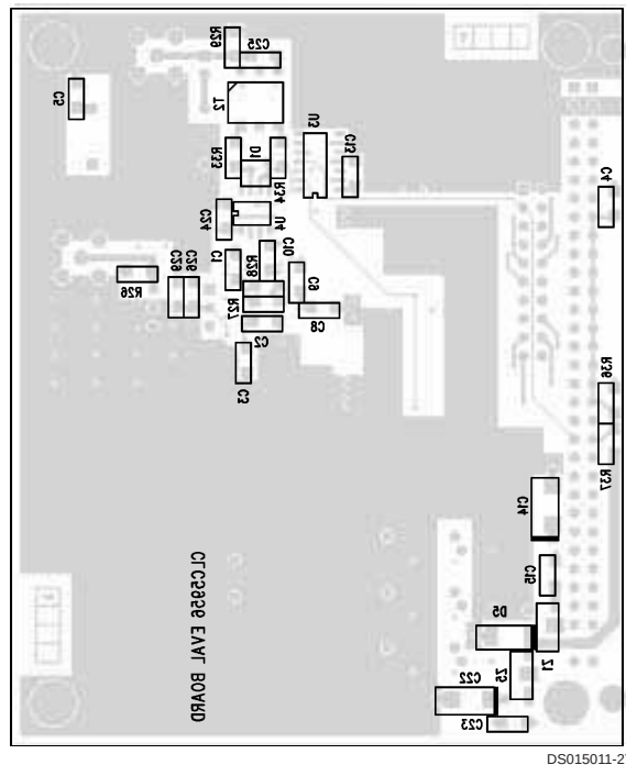
CLC730079 Layer 4
