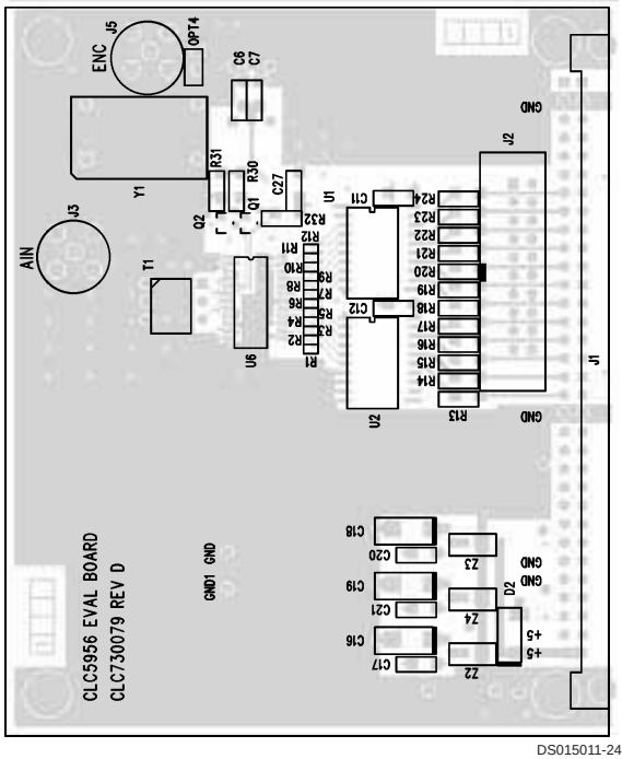
CLC730079 Layer 1
