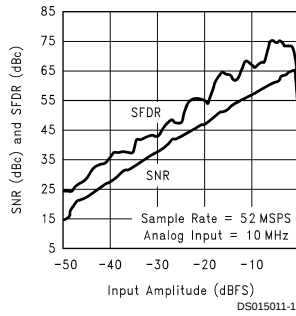
SNR and SFDR vs Input Amplitude
