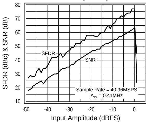
SFDR & SNR vs. Input Amplitude
