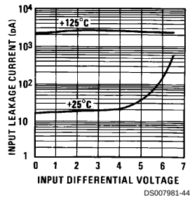
Input Leakage
