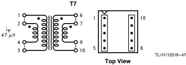
FIGURE 27. Schott 26606
