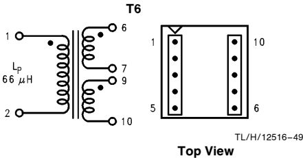
FIGURE 28. Schott 67140900
