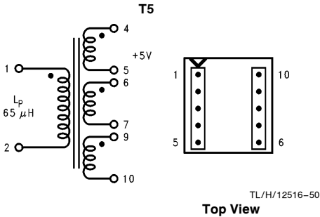
FIGURE 29. Schott 67140890
