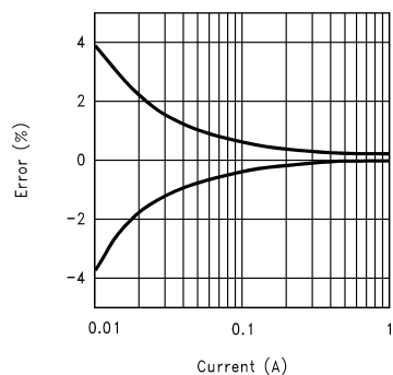
Error vs Current (LM3814-1.0 and LM3815-1.0) (Note 10)
