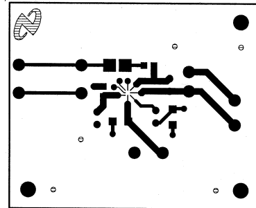
Top Layer
