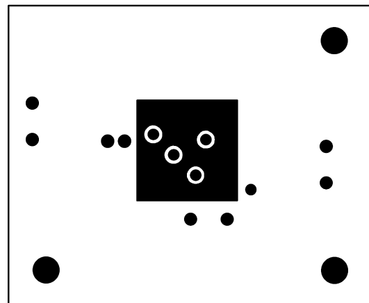
Inner Layer V DD
