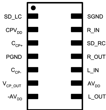
LLP Package
