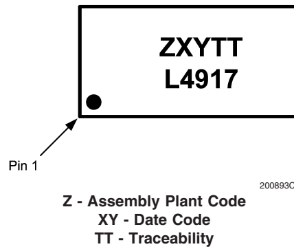
LLP Marking
