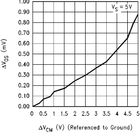
\Delta V_{OS} vs \Delta V_{CM}
