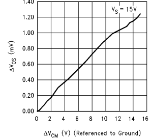
\Delta V_{OS} vs \Delta V_{CM}
