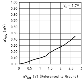
\Delta V_{OS} vs \Delta V_{CM} V_S = 2.7V
