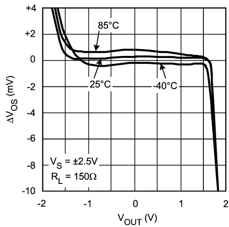
\Delta V_{OS} vs. V_{OUT}
