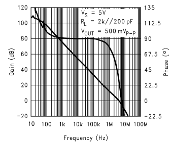
Gain/Phase
