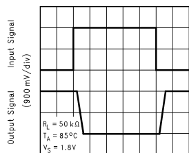
Time (10 \mu s /div) DS100979-D7
